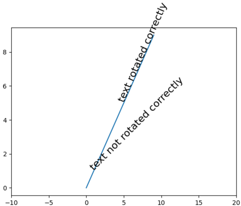
Fig. 2: Example of the new transform_rotates_text parameter
